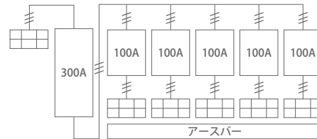
分電盤 300A
