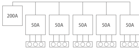
分電盤 200A
