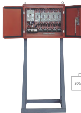
分電盤 200A
