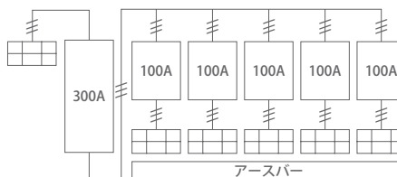
分電盤 300A
