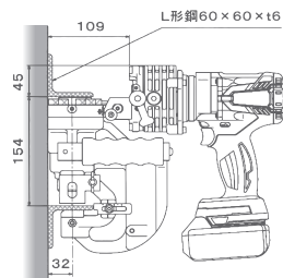
壁からの穴あけ寸法図【単位mm】 (HPC-N188WBL)
